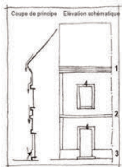
1 : Corniche 2 : Larmier 3 : Soubassement 4 : encadrements de baies
