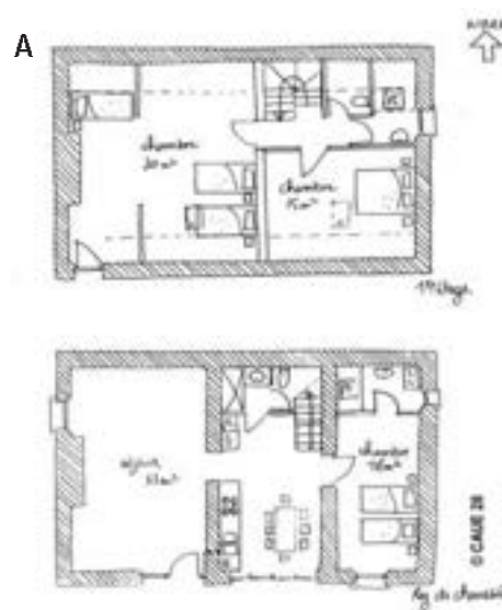
La solution (A) : aménagement d'un gîte comportant trois chambres.
