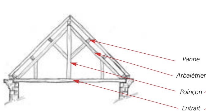
Ferme classique avec poinçon sur l'entrait
